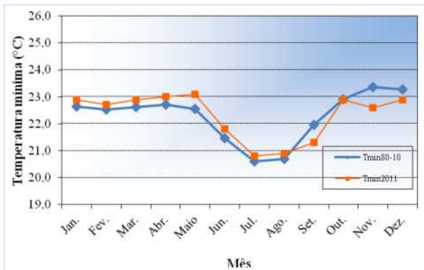
Figura 2. Valores médios mensais da temperatura mínima do ar referentes a 2011 e ao período de 1980 a 2010. Teresina, PI.
