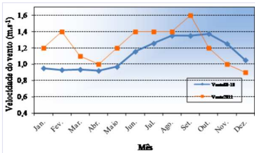
Figura 5. Valores médios mensais da velocidade do vento referentes a 2011 e ao período de 1980 a 2010. Teresina, PI.
