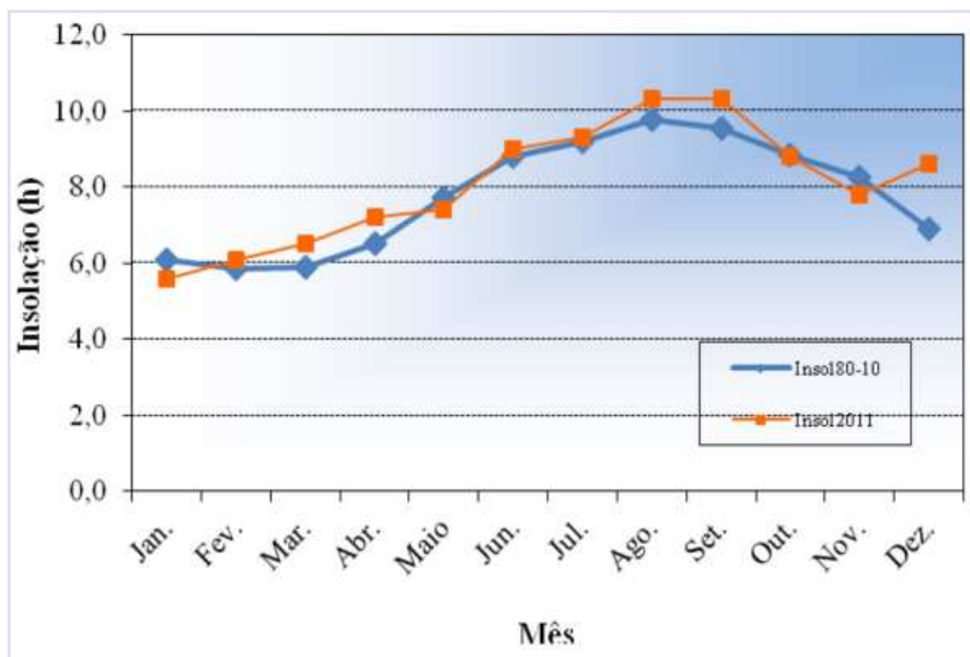
Figura 6. Valores médios mensais da insolação referentes a 2011 e ao período de 1980 a 2010. Teresina, PI.
