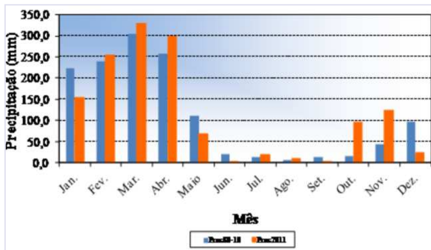
Figura 8. Totais mensais da precipitação pluviométrica referentes a 2011 e valores médios dos totais mensais da precipitação pluviométrica referentes ao período de 1980 a 2010. Teresina, PI.
