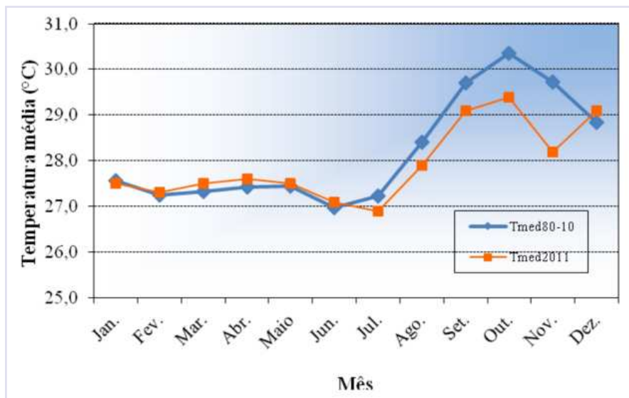
Figura 3. Valores médios mensais da temperatura média do ar referentes a 2011 e ao período de 1980 a 2010. Teresina, PI.
