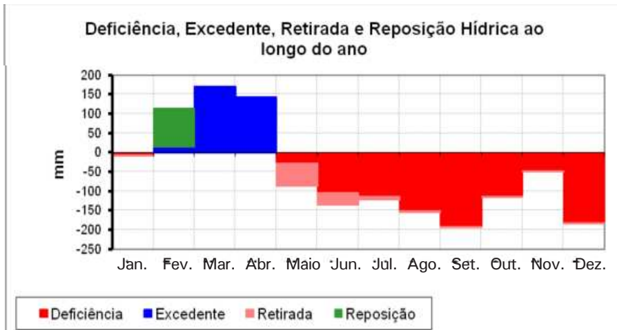
Figura 10. Extrato do balanço hídrico para o município de Teresina, PI, no ano de 2011.
