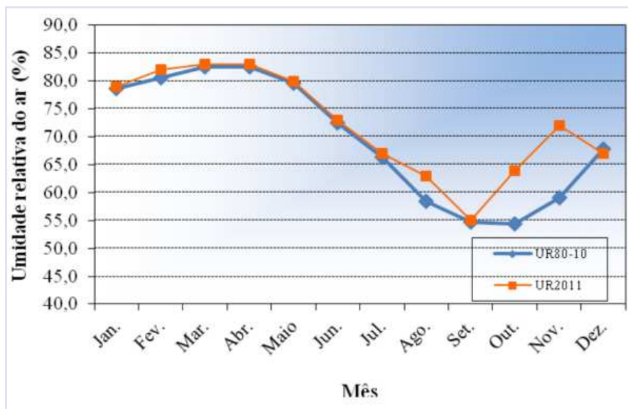
Figura 4. Valores médios mensais da umidade relativa do ar referentes a 2011 e ao período de 1980 a 2010. Teresina, PI.
