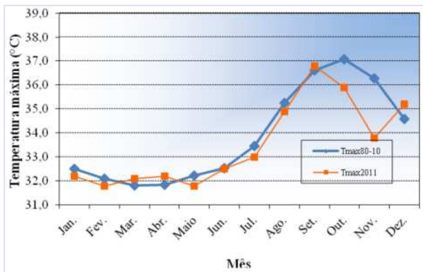
Figura 1. Valores médios mensais da temperatura máxima do ar referentes a 2011 e ao período de 1980 a 2010. Teresina, PI.
