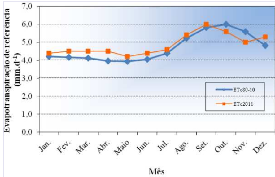
Figura 7. Valores médios mensais da evapotranspiração de referência (ETo) pelo método de Penman-Monteith referentes a 2011 e ao período de 1980 a 2010. Teresina, PI.
