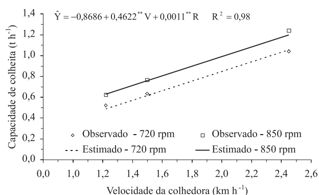
FIGURA 4. Capacidade de colheita da colhedora em função da velocidade de deslocamento (V) e rotação do cilindro trilhador (R).
