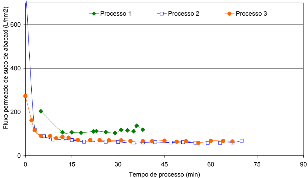
Fig. 2. Fluxo permeado de suco de abacaxi ao longo do tempo de processamento das membranas de microfiltração ( \Delta P = 1 Bar)
