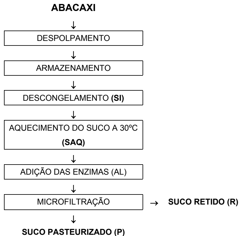
Fig. 1. Fluxograma do processo de pasteurização de suco de abacaxi.
