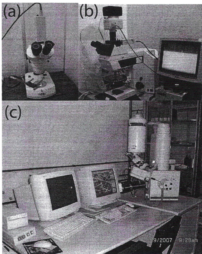
Fig. 1. Equipamentos de microscopia utilizada: (a) Lupa; (b) Microscópio Ótico com Luz Polarizada; © FEG-MEV.
