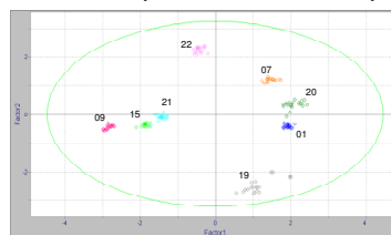
Figura 1. PCA dos resultados analíticos quantitativos obtidos pelos métodos de referência
