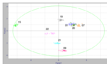
Figura 2. PCA dos dados qualitativos de reflectâncias obtidos por NIRS.
