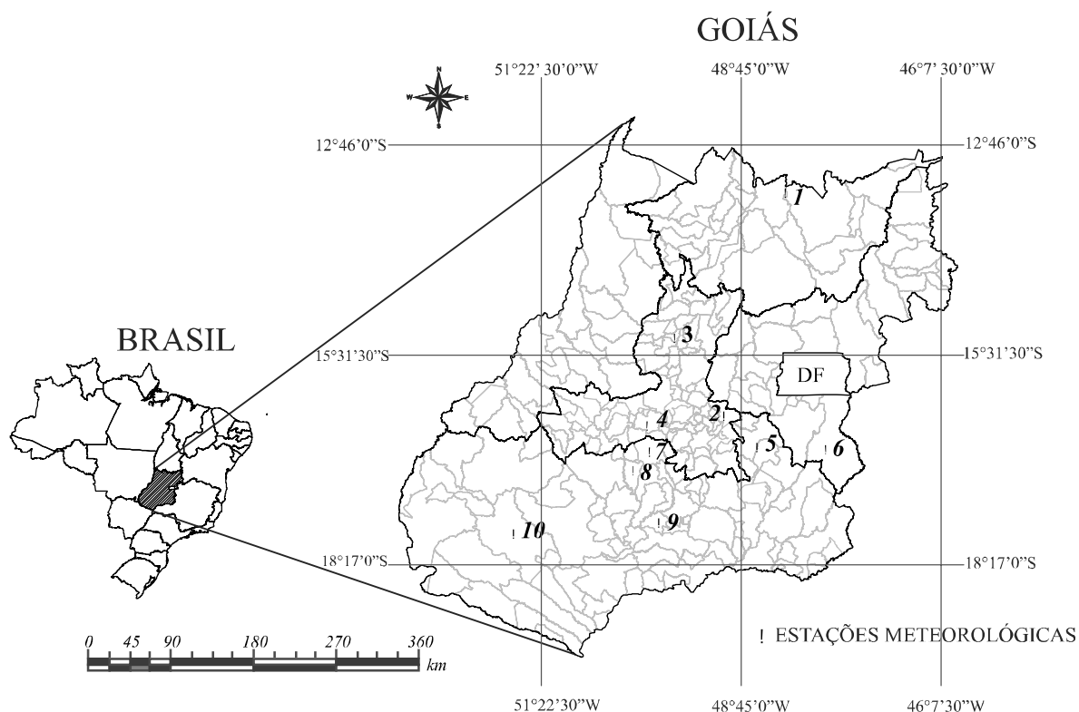
Figura 1 - Mapa com a localização geográfica das estações meteorológicas utilizadas no estudo. Números representam as IDs das estações meteorológicas
