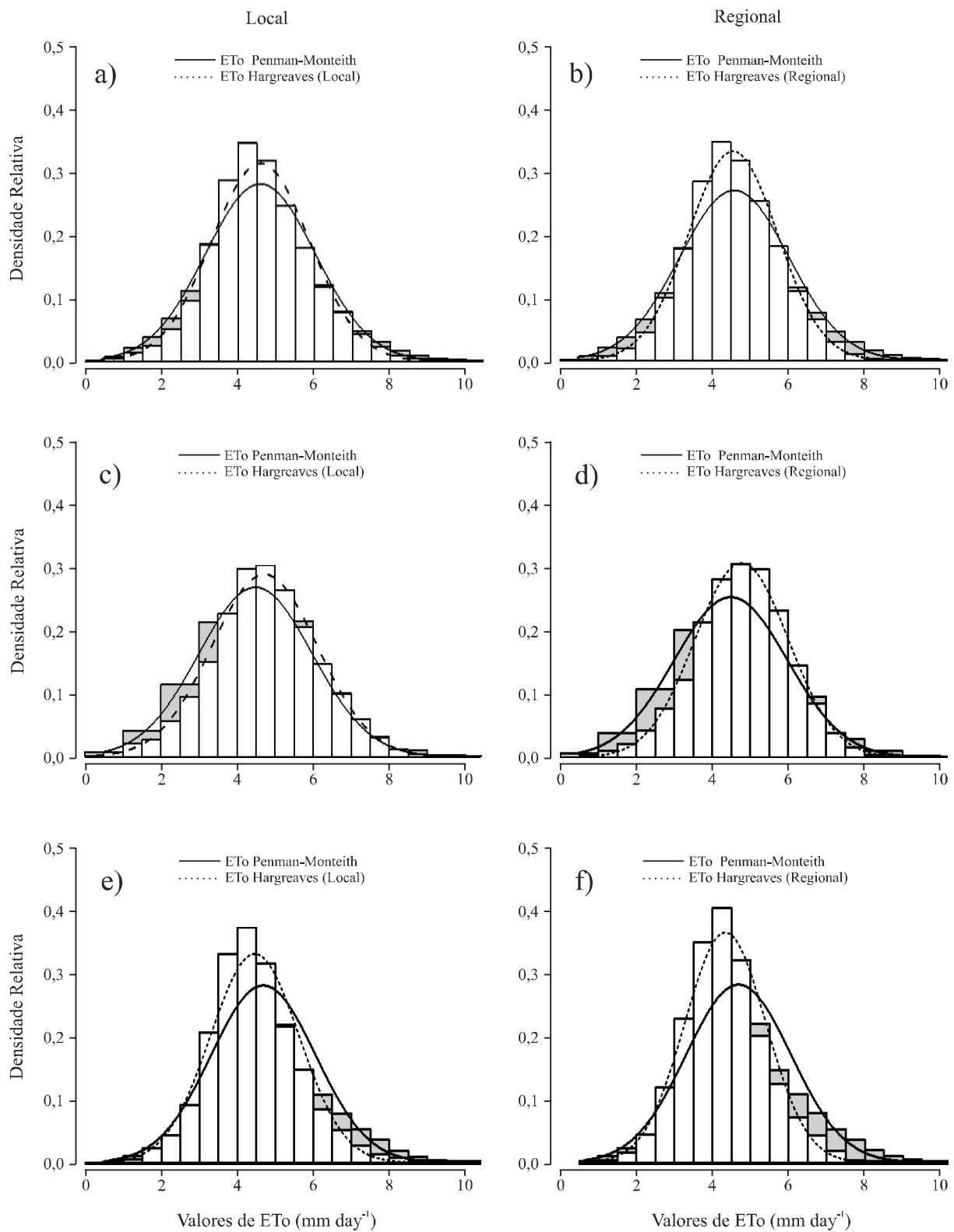
Figura 2 - Densidade relativa e histograma de frequência (branco - Hargreaves, cinza - Penman-Monteith) dos valores de ETo estimado por Hargreaves e Penman-Monteith pelo processo local e regional (a e b) considerando-se todos os meses da serie histórica de dados das 10 estações meteorológicas; (c e d) considerando-se somente os meses chuvosos (outubro a março); e (e e f) considerando-se somente os meses secos(abril a setembro)
