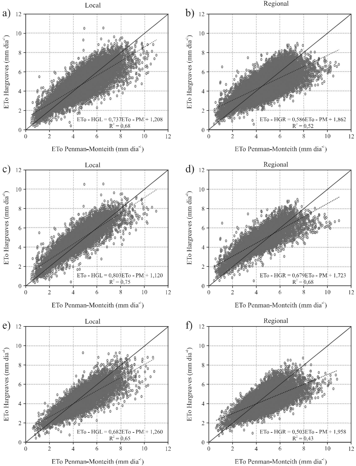
Figura 3 - Regressão entre a evapotranspiração de referência (ET o ) estimada pela equação de Hargreaves e Penman-Monteith. (a e b) considerando-se todos os meses da serie histórica de dados das 10 estações meteorológicas; (c e d) considerando-se somente os meses chuvosos (outubro a março); e (e e f) considerando-se somente os meses secos (abril a setembro). Linha de regressão (tracejada) e linha 1:1 (contínua)
