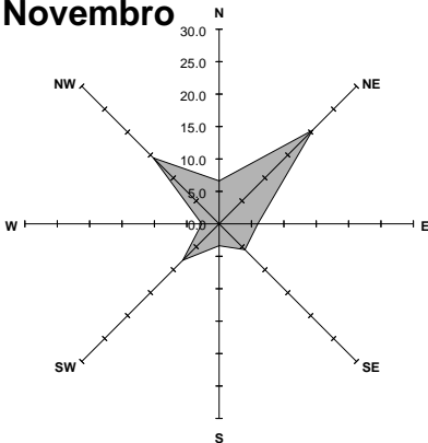
Fig. 6. Frequência média da direção dos ventos na região de Dourados nos meses de julho a dezembro.
