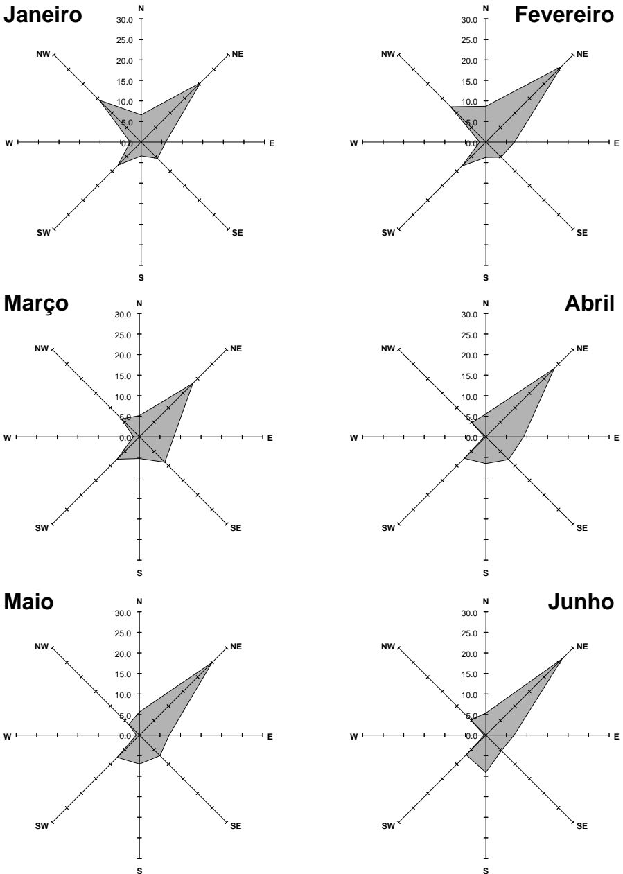
Fig. 5. Frequência média da direção dos ventos na região de Dourados nos meses de janeiro a junho.
