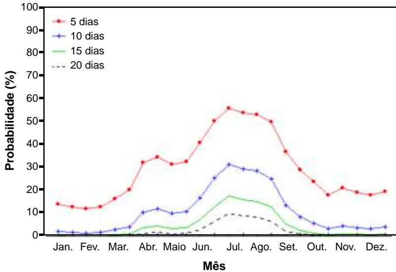
Fig. 8. Probabilidade de ocorrência de dias sem chuva com, no mínimo, 5, 10, 15 e 20 dias na região de Dourados.
