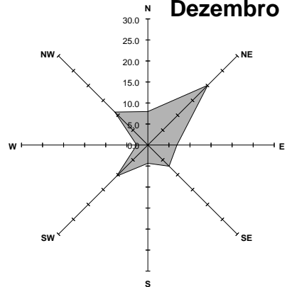
Fig. 6. Frequência média da direção dos ventos na região de Dourados nos meses de julho a dezembro.
