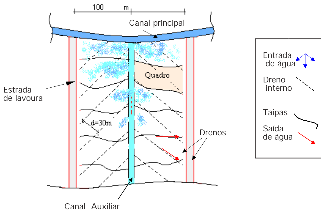
Fig. 1. Planejamento de área não sistematizada para irrigação por inundação intermitente em culturas alternativas ao arroz em várzea.
