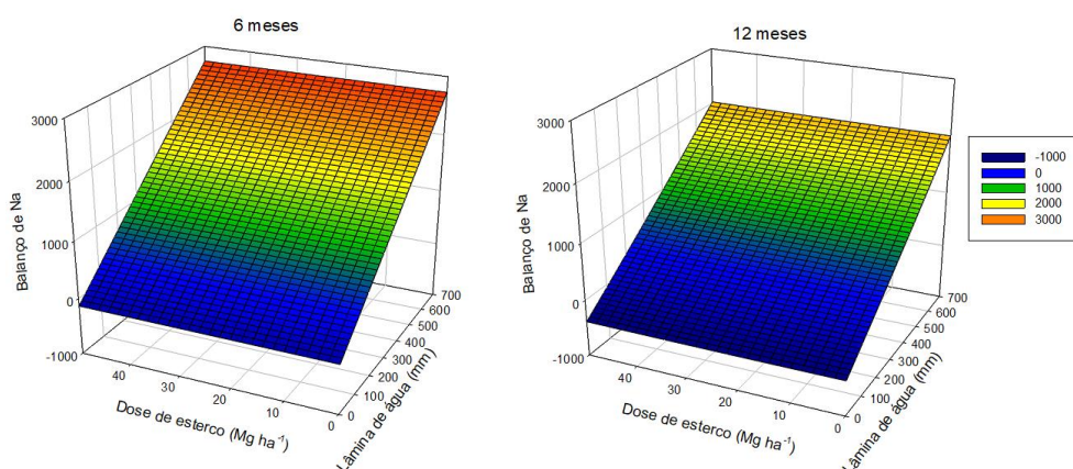
Figura 7. Balanço de \text{Na}^+ de acordo com lâminas de água no plantio de palma forrageira aos seis e doze meses no estudo da palma forrageira na área experimental da Embrapa Semiárido (Petrolina/PE).
