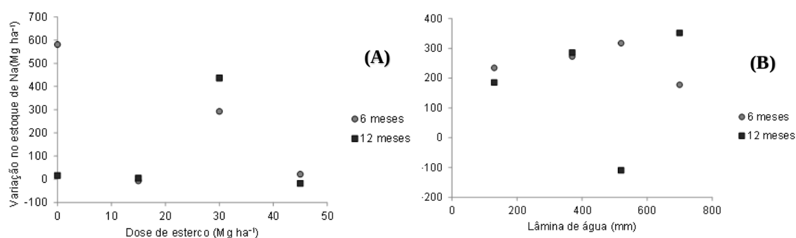
Figura 4. Variação dos estoques de \text{Na}^{+} de acordo com doses de esterco (A) e lâminas de água (B) aos seis e doze meses no estudo da palma forrageira na área experimental da Embrapa Semiárido (Petrolina/PE).
