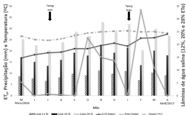
Figura 1 – Evapotranspiração de referência, precipitação (mm), temperatura °C e lâminas de água [12%, 20% e 28% ( ET_0 )] de maio de 2016 a abril de 2017 no período de estudo da palma forrageira na área experimental da Embrapa Semiárido (Petrópolis/PE).
