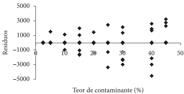
Figura 8. Resíduos do ajuste na verificação de linearidade em café em pó segundo teor (%) do contaminante (milho).
