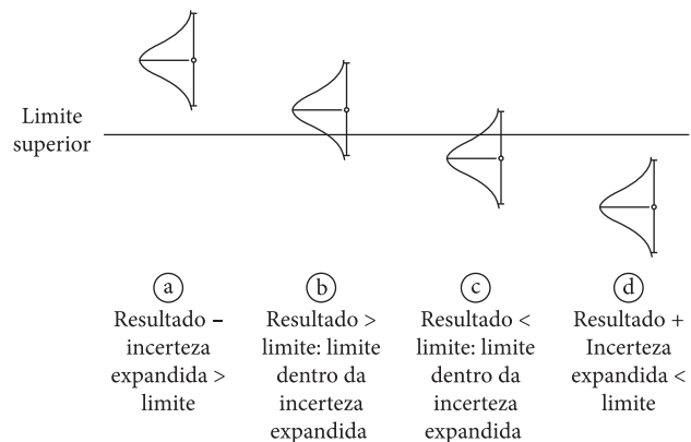
Figura 2. Cenários da verificação de conformidade com limite de especificação do tipo “superior a”. Fonte: Ellison e Williams (2007).
