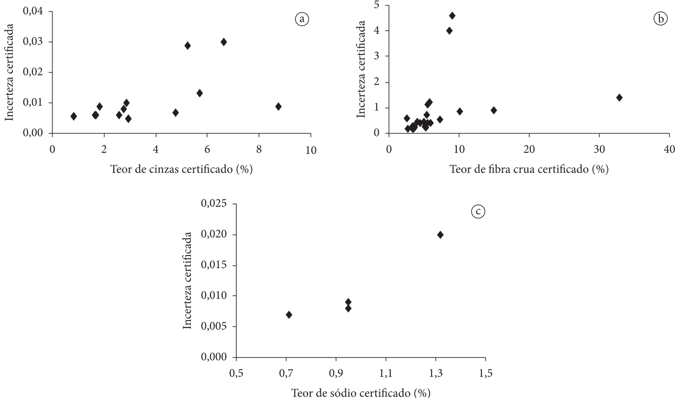
Figura 4. Incertezas certificadas em função de teores certificados de medições de a) cinzas; b) fibra crua; e c) sódio em ensaios FAPAS de proficiência.
