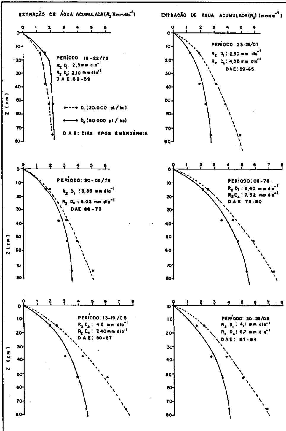
FIG. 4. Valores acumulados de extração de água ( R_z ), em função da profundidade ( Z ) e densidade de plantio, em diferentes períodos, durante o desenvolvimento da cultura.
