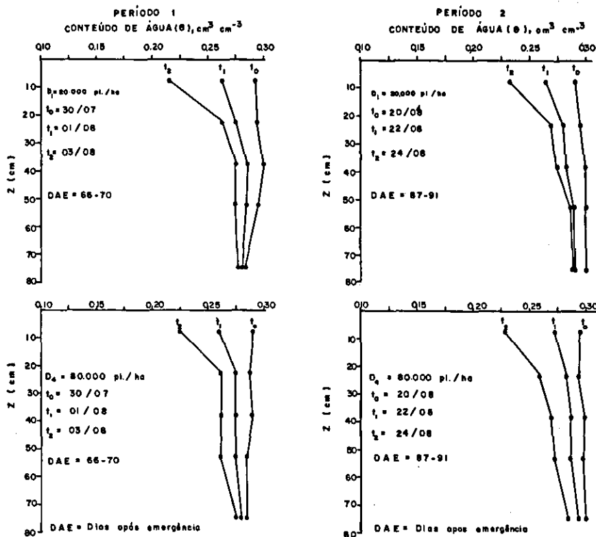
FIG. 1. Variação dos conteúdos de água do solo ( \theta ), em função da profundidade ( z ) e densidade de plantio, em duas épocas, durante o desenvolvimento da cultura.
