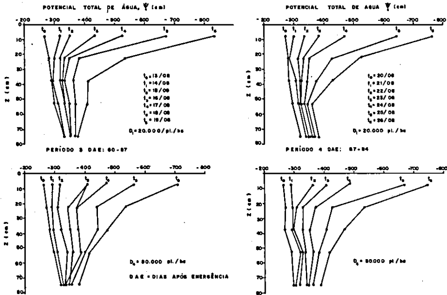
FIG. 2. Variação do potencial total de água no solo ( \psi ), em função da profundidade ( z ) e densidade de plantio, em dois períodos (1 e 2), durante o desenvolvimento da cultura.
