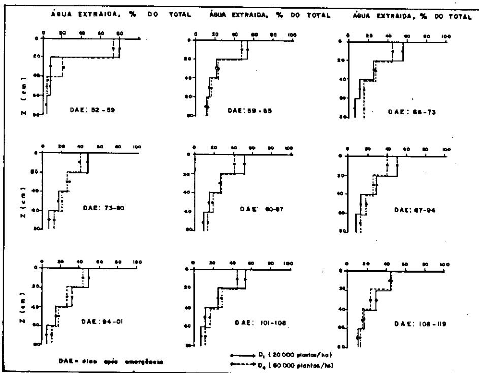
FIG. 6. Variação da água extraída (% do total), em função da profundidade e densidade de plantio, em diferentes períodos, durante o desenvolvimento da cultura.
