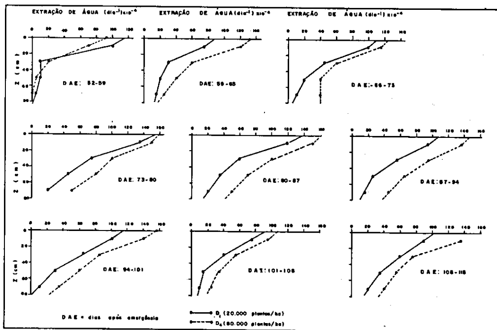
FIG. 5. Extração de água do solo, em função da profundidade e densidade de plantio, em diferentes períodos, durante o desenvolvimento da cultura.
