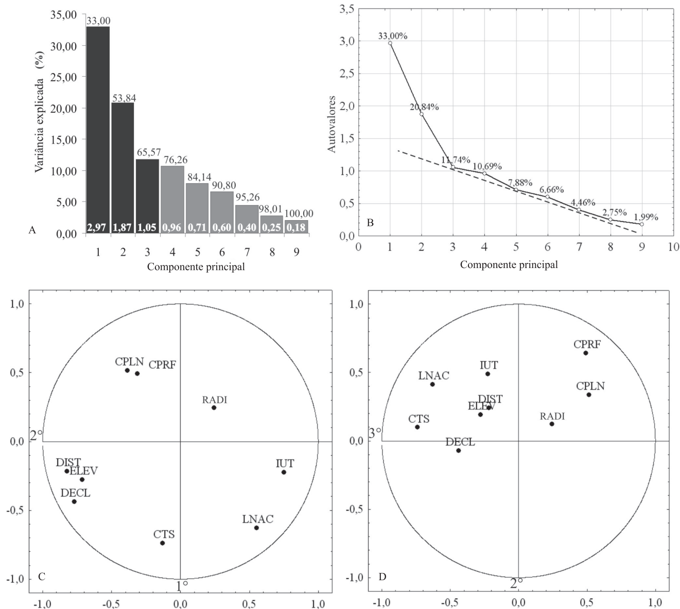
Figura 2. Variância explicada pelas nove componentes principais (CP) geradas (A), "Scree plot" (B), diagramas de dispersão circular (C e D). ELEV, elevação; DECL, declividade; CPLN, curvatura planar; CPRF, curvatura de perfil; DIST, distância à drenagem; RAD, radiação relativa disponível; LNAC, área de contribuição; IUT, índice de umidade topográfica; e CTS, capacidade de transporte de sedimento. Autovalores de cada componente constam em branco na base e no interior de cada barra. As três primeiras barras em negrito possuem autovalor maior do que a unidade. Valor sobre as barras indica o percentual de variância acumulada.
