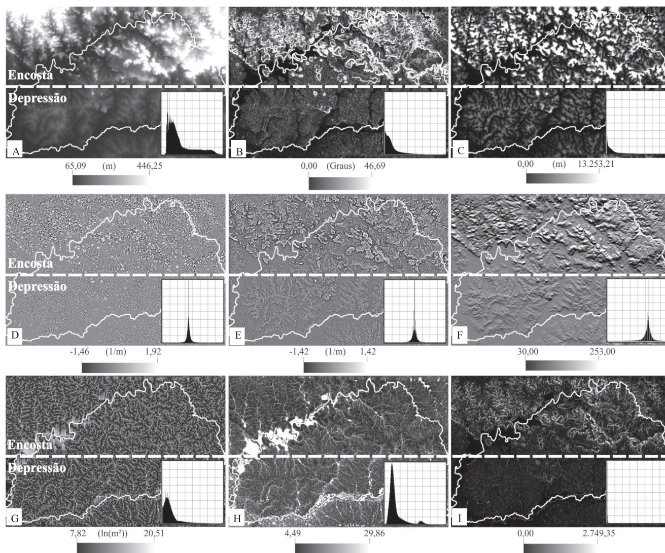
Figura 1. Distribuição espacial dos atributos do terreno (e seus histogramas), na área de estudo: A, elevação (ELEV); B, declividade (DECL); C, distância à drenagem (DIST); D, curvatura planar (CPLN); E, curvatura de perfil (CPRF); F, radiação relativa disponível (RADI); G, área de contribuição (LNAC); H, índice de umidade topográfica (IUT); I, capacidade de transporte de sedimento (CTS). Nas figuras, a área superior está localizada na Encosta do Planalto e a parte inferior na Depressão Central.
