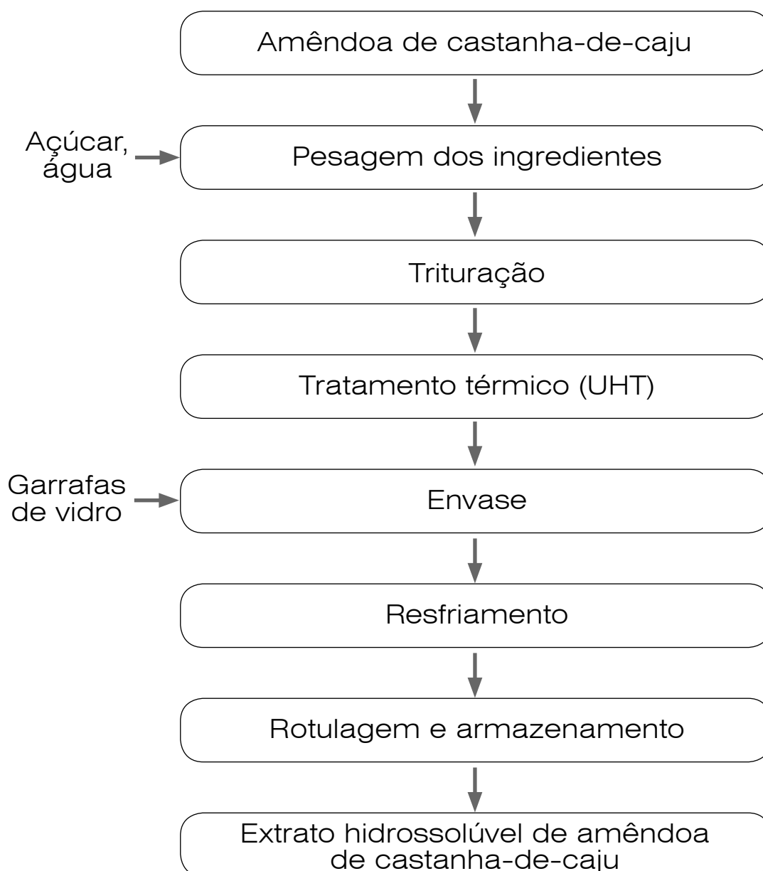
Figura 1. Fluxograma do processo para obtenção do extrato hidrossolúvel de amêndoa de castanha-de-caju.
