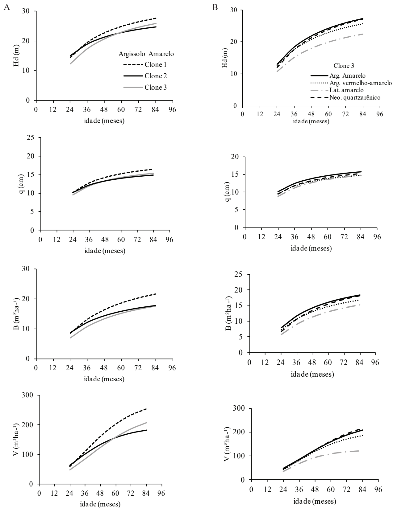
Figura 2. Curva de crescimento em altura dominante (Hd), em m, diâmetro quadrático (q), em cm, área basal, em \text{m}^2\text{ha}^{-1} e volume de madeira, \text{m}^3\text{ha}^{-1} para os três clones no Argissolo Amarelo (A) e o clone 3 nos diferentes tipos de solo (B) em função da idade.
