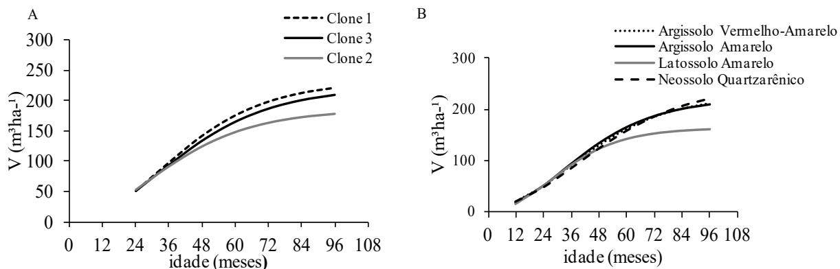
Figura 3. Modelo de Gompertz com inclusão de precipitação pluviométrica. (A) Curvas de produção, dos diferentes clones no Argissolo Amarelo, e (B) do clone 3 nos diferentes tipos de solo, considerando a precipitação média de 1.083 mm.
