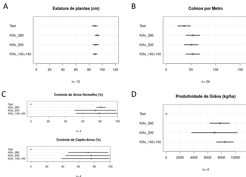
Figura 1. (A) densidade de perfílios (colmos por metro); (B) estatura de plantas (cm); (C) controle de arroz-vermelho e capim-arroz (%); e (D) produtividade de grãos de arroz-irrigado, linhagem precoce CL (Inta Puitá CL x BRS Pampa), em função de tratamento herbicida e momento de aplicação.
