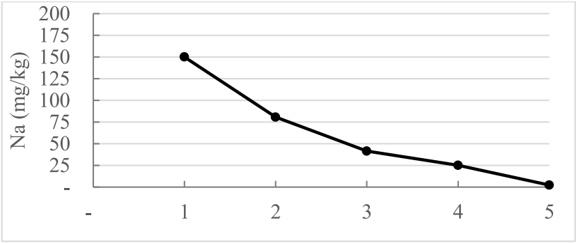
Figura 8 – Variação no Na e Ca trocáveis em amostras coletadas no solo remineralizado, em experimento de campo (adaptado de Silva,2016).
