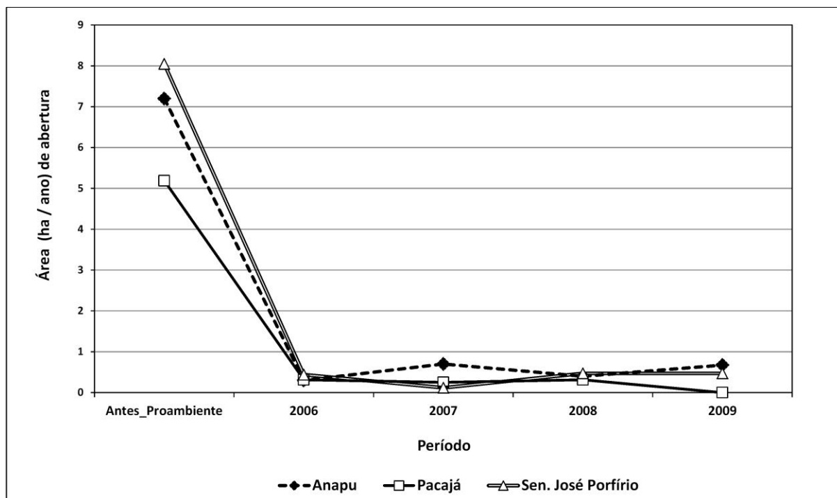
Figura 02 - Média anual de área aberta em floresta primária (ha) em propriedades rurais antes e pós PROAMBIENTE, polo transamazônica, região do Xingu, Estado do Pará.
