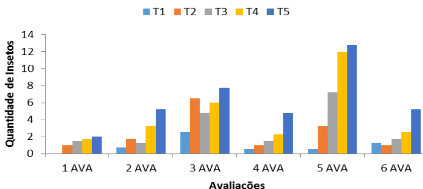
Figura 1. Valores da quantidade de ninfas de cigarrinhas encontradas durante as seis avaliações. Os tratamentos são: T1 – 0% de palhada, T2 – 25% de palhada, T3 – 50% de palhada, T4 – 75% de palhada e T5 – 100% de palhada. As avaliações são: 1 AVA – 7 dias, 2 AVA – 15 dias, 3 AVA – 30 dias, 4 AVA – 60 dias, 5 AVA – 90 dias, 6 AVA – 120 dias.
