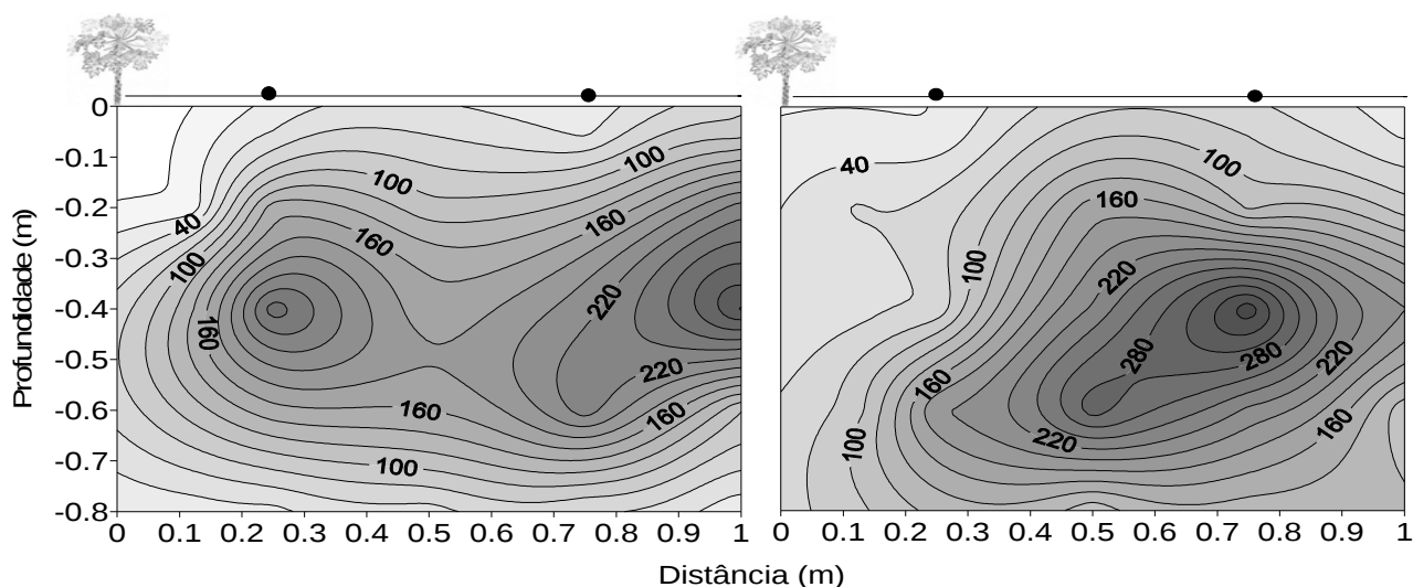
Figura 3 - Água disponível para T1 – gotejamento com quatro emissores de 4 \text{ L h}^{-1} por planta em uma linha lateral (A) e T2 – oito emissores de 4 \text{ L h}^{-1} por planta em duas linhas laterais (B), seis horas após a irrigação.
