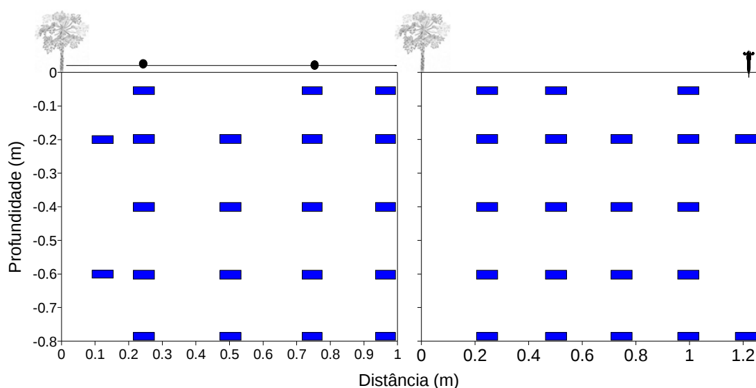
Figura 1 - Posição das sondas de TDR no perfil de solo para os tratamentos irrigados por gotejamento (A) e microaspersão (B).
