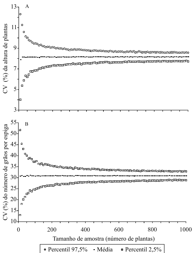
Figura 2. Percentil 2,5%, média e percentil 97,5% das mil estimativas do coeficiente de variação (CV) de: A, altura de plantas; e B, número de grãos por espiga, para os tamanhos de amostra n = 10, 20, \dots, 1.000 plantas, no híbrido triplo DKB566, avaliado na safra 2008/2009.
