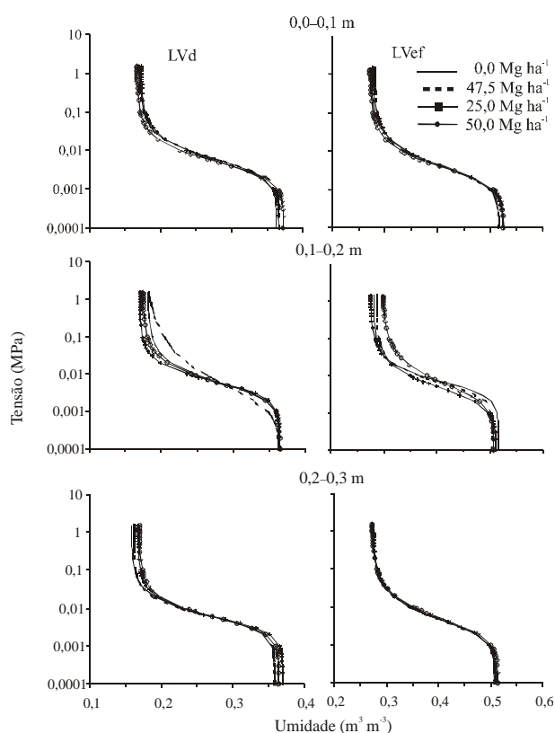
Figura 1. Curvas de retenção de água em diferentes doses de biofóssido e camadas de Latossolo Vermelho distrófico, textura média (LVd), e Latossolo Vermelho eutroférico argiloso (LVef).
