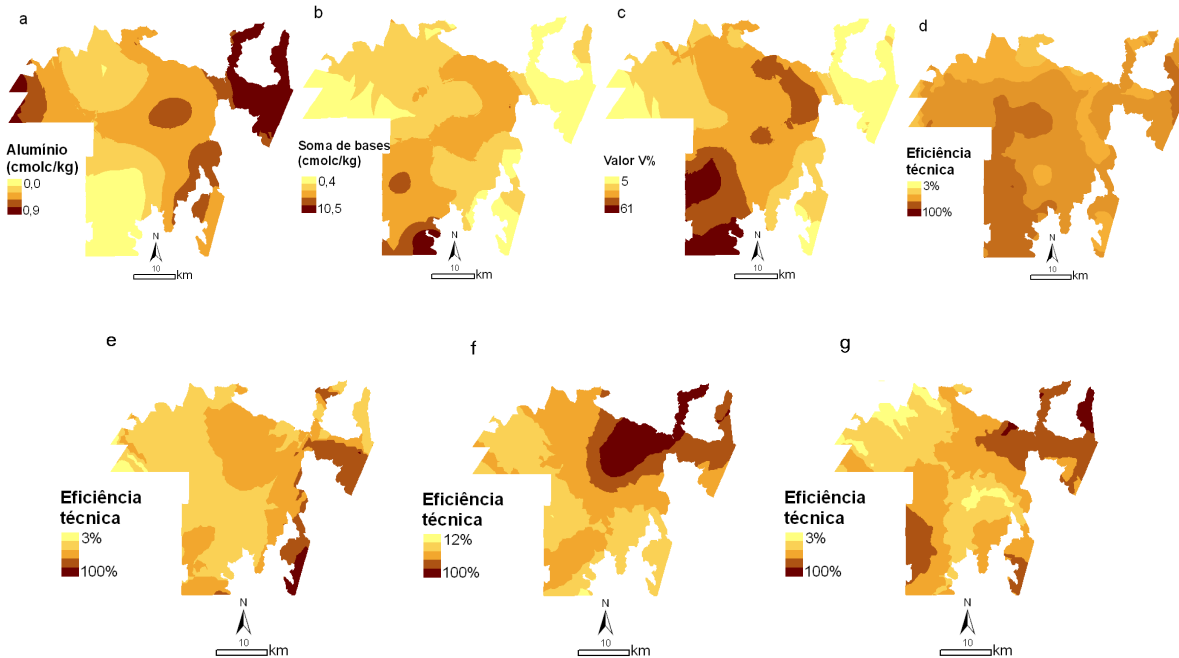
Figura 1. Distribuição espacial por krigagem dos teores de alumínio (a), soma de bases (b), V% (c), eficiência técnica para a cultura do arroz (d), do feijão (e), do milho (f) e do café (g).
