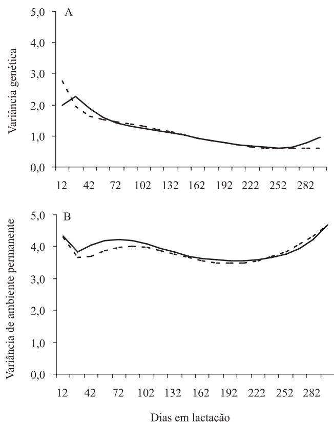
Figura 2. Estimativas médias posteriores de variâncias genética (kg 2 ) (A) e de ambiente permanente (kg 2 ) (B), para os modelos AS-4 (—) e W025-6 (- - -), ao longo da lactação de bovinos da raça Gir leiteira entre 1990 e 2007.
