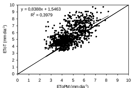
Figura 2. Regressão linear entre os valores de ETo calculados pelos métodos de Thornthwaite (EToT) e Penman-Monteith (EToPM), na escala decendial.
