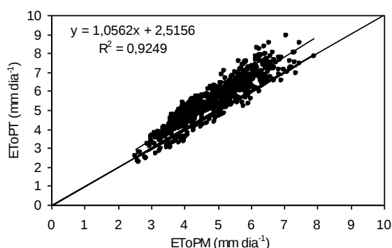
Figura 1. Regressão linear entre os valores de ETo calculados pelos métodos de Priestley-Taylor (EToPT) e Penman-Monteith (EToPM), na escala decendial.
