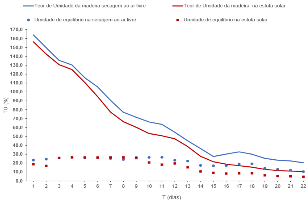
Figura 5. Curvas resultantes dos processos de secagem em estufa solar e ao ar livre.
