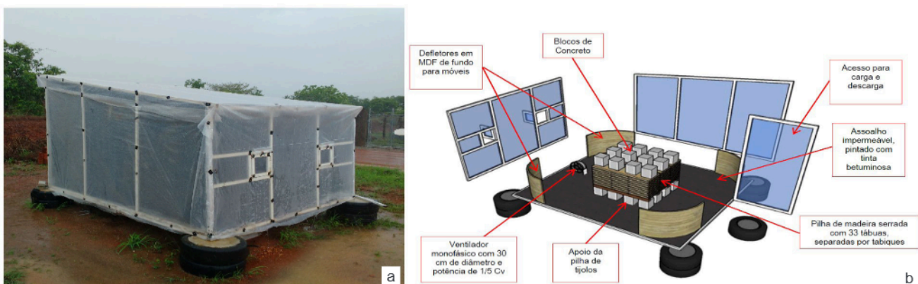
Figura 2. Estufa de secagem solar instalada nas adjacências do Laboratório de Tecnologia e Utilização de Produtos Florestais da Universidade Federal do Tocantins (UFT), no município de Gurupi, Tocantins.
