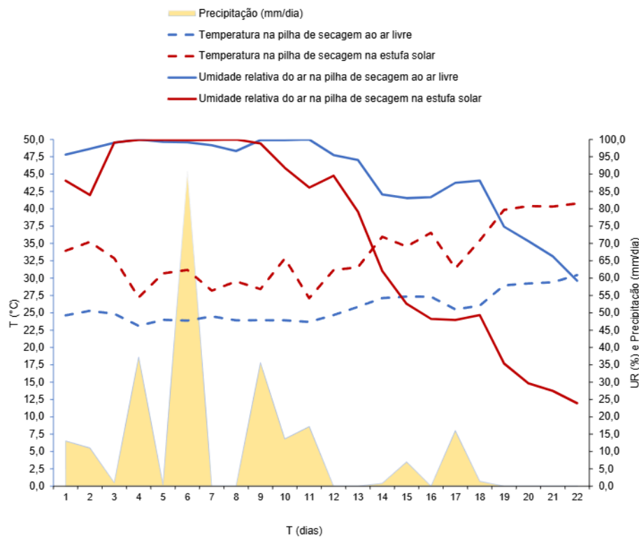
Figura 4. Variáveis ambientais coletadas nos processos de secagem solar em estufa e ao ar livre. Figure 4. Environmental variables collected in greenhouse and outdoor solar drying processes.
