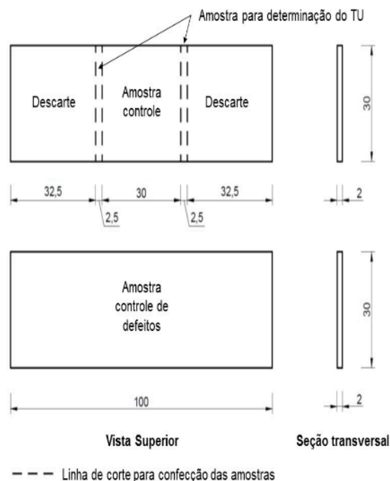
Figura 1. Dimensionamento das amostras utilizadas na secagem ao ar livre e na secagem em estufa solar. Figure 1. Sizing of samples used in outdoor drying and drying in a solar kiln.
