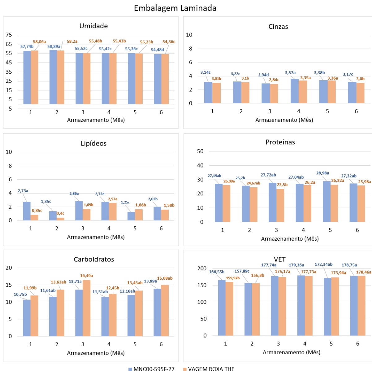
Figura 1. Composição centesimal dos grãos imaturos branqueados e congelados dos genótipos de feijão-caupi conservados em embalagem laminada em seis meses de armazenamento (base seca). Teresina/PI, 2022. Médias com letras iguais no mesmo genótipo ao longo dos meses de armazenamento não diferem entre si pelo teste Tukey ( p < 0,05 ).
