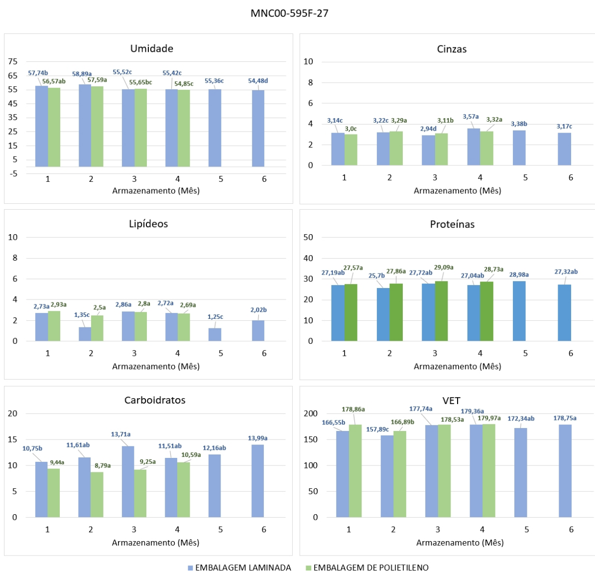
Figura 2. Composição centesimal dos grãos imaturos branqueados e congelados da linhagem MNC00-595F-27 conservada em embalagem laminada e de polietileno em seis e quatro meses de armazenamento, respectivamente (base seca). Teresina/PI, 2022. Médias com letras iguais na mesma embalagem ao longo dos meses de armazenamento não diferem entre si pelo teste Tukey ( p < 0,05 ).
