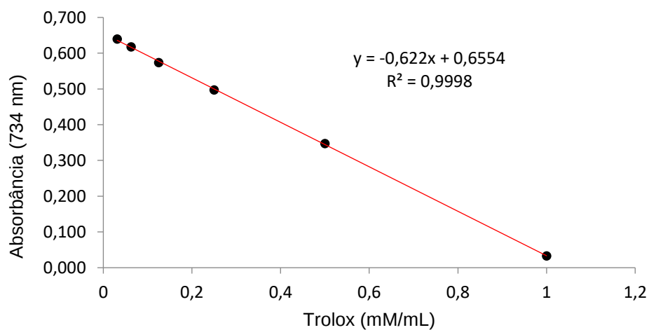
Anexo 2. Curva de calibração-resposta de inibição do radical ABTS •+ frente ao padrão Trolox®.
