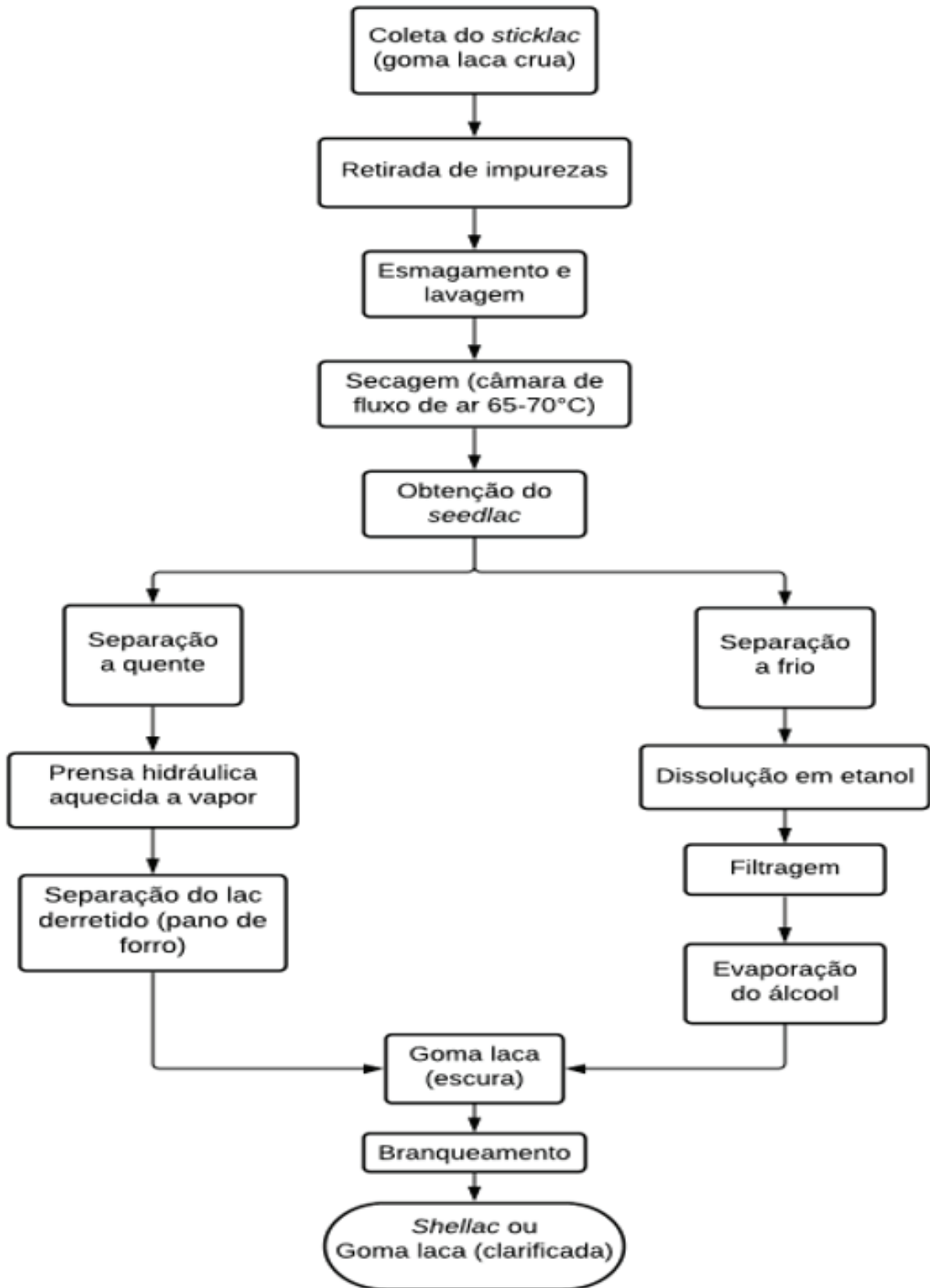
Figura 2. Fluxograma do processamento para obtenção da goma-laca ( shellac ).
