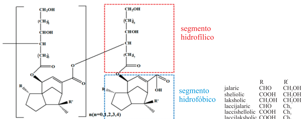
Figura 1. Estrutura geral da molécula anfifílica de goma-laca.
