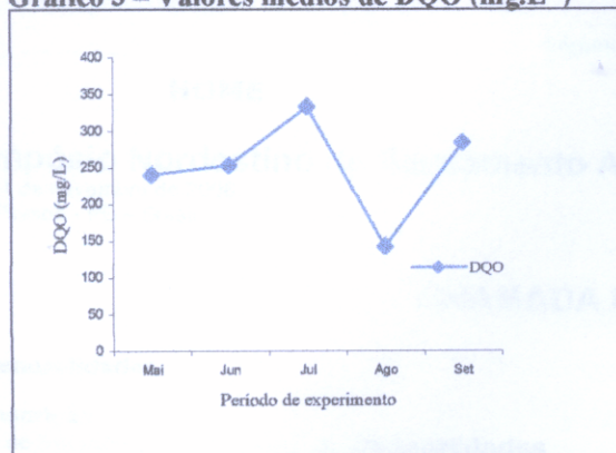
Gráfico 3 – Valores médios de DQO ( \text{mg.L}^{-1} )
