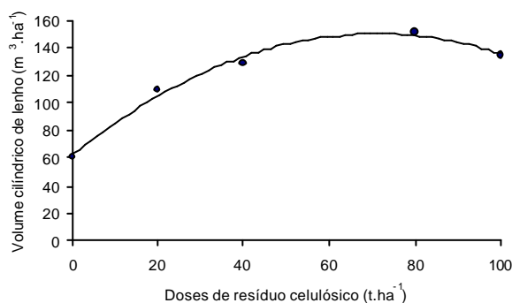
FIGURA 2. Volume cilíndrico de lenho de árvores de Pinus taeda L., aos 7 anos de idade, em função da aplicação de doses de resíduo celulósico.
