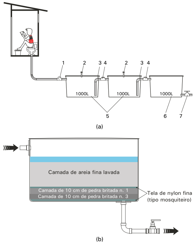
Figura 1 Esquema da fossa biodigestora. a) todo o sistema e b) 3ª. caixa projetada para remoção da matéria orgânica.
