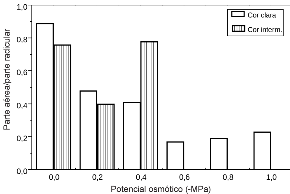
FIG. 2. Proporção parte aérea/parte radicular de plântulas de algarobeira após sete dias de permanência em soluções PEG 6000, com diferentes potenciais osmóticos.
