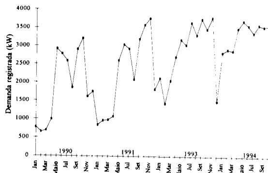
FIG. 1. Comportamento da demanda registrada durante o quadriênio analisado (1990-93), na agroindústria de processamento de cana.
