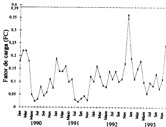
FIG. 2. Comportamento do fator de carga durante o quadriênio analisado (1990-93), na agroindústria de processamento de cana.
