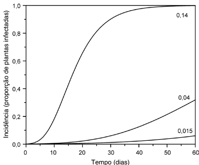
Fig. 1. Curvas de progresso de doença estimadas pelo modelo de Gompertz, com três taxas de progresso da doença: 0,015, 0,04 e 0,14. O inóculo inicial ( y_0 ) foi fixado em 0,001 e a assíntota ( y_{max} ), em 1 para as três curvas.
