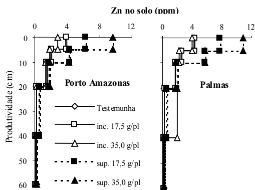
FIG. 1. Efeito da aplicação de Zn no solo no teor de Zn extraído com HCl 0,1 N.
