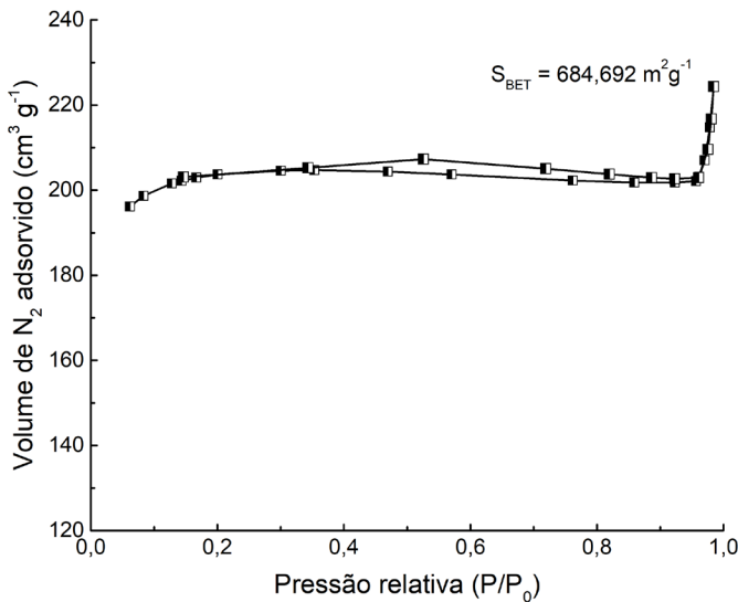
Figura 1. Isotermas de adsorção/dessorção de nitrogênio (N 2 ), a 77 K, para o carvão ativado de bambu (CAB). S_{\text{BET}} = área superficial BET.
