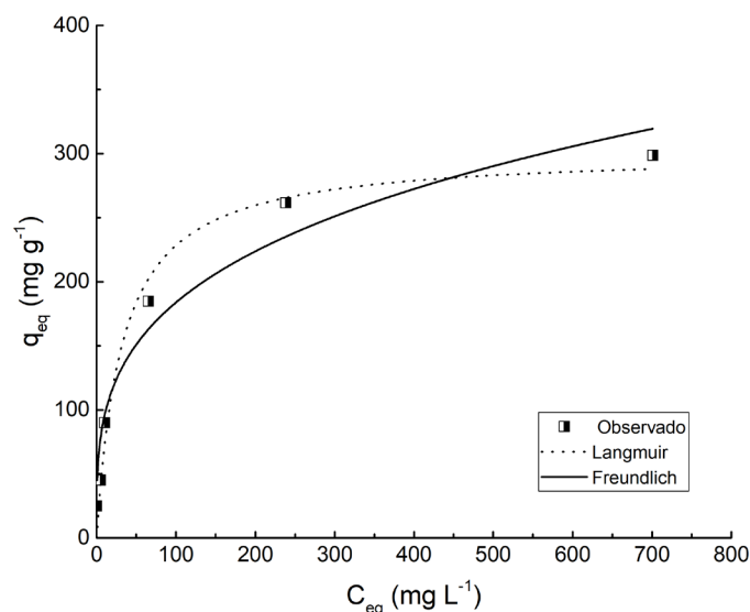
Figura 3. Isoterma de adsorção do azul de metileno (AM) pelo CAB.
