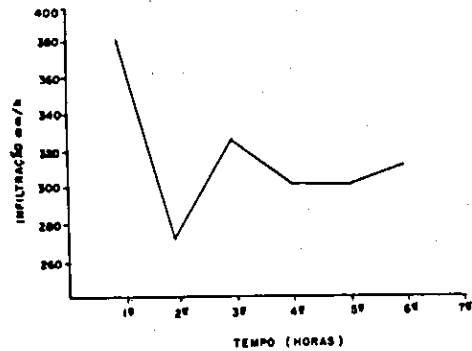
FIG. 24. Capacidade de infiltração do perfil n.º 13.
