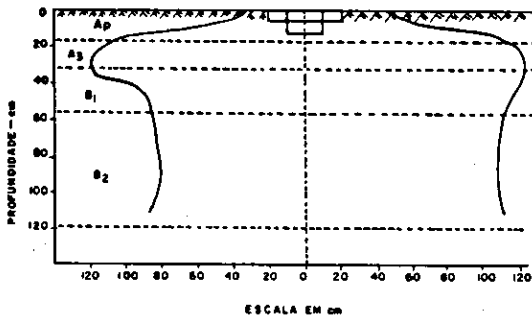
FIG. 21. Umedecimento do solo do perfil n.º 8.
