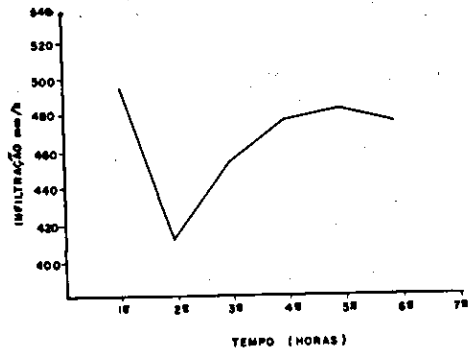
FIG. 23. Capacidade de Infiltração do perfil n.º 15.
