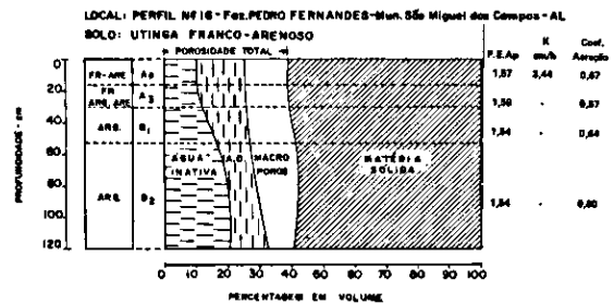
FIG. 4. Diagrama físico-volumétrico do perfil nº 16.
