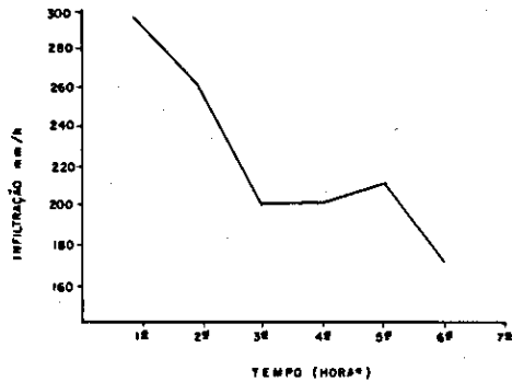
FIG. 25. Capacidade de infiltração do perfil n.º 3.
