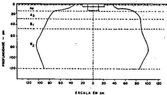
FIG. 22. Umedecimento do solo do perfil n.º 7.
