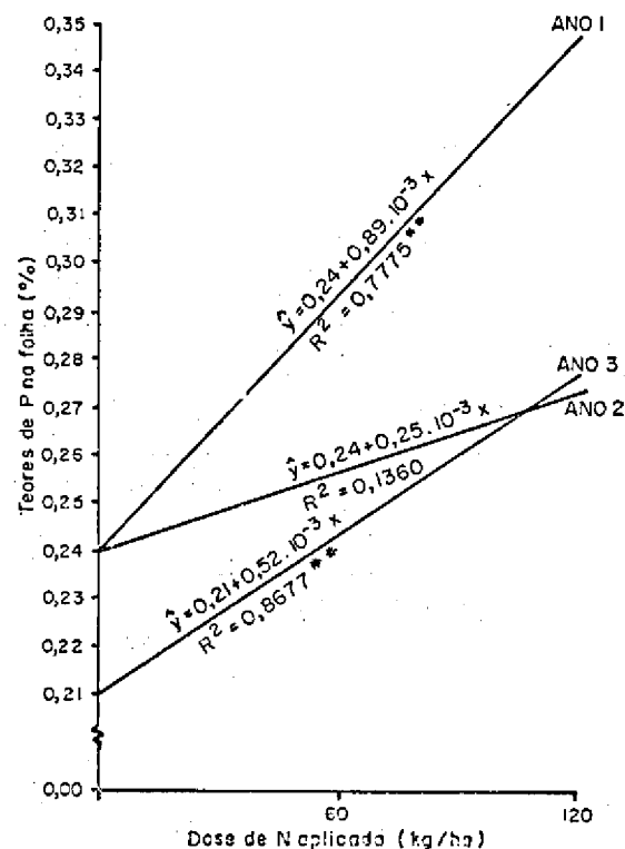
Fig. 2. Efeito da adubação nitrogenada na absorção de P.
