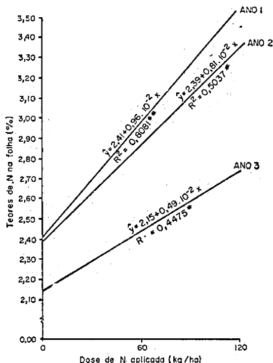
FIG. 1. Efeito da adubação nitrogenada na absorção de
