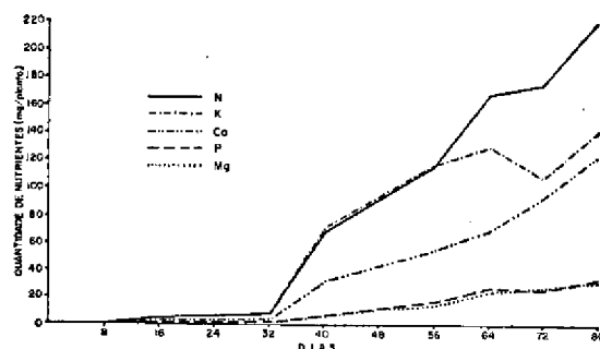
FIG. 2. Curva de absorção total de nutrientes de acordo com a época de amostragem.
