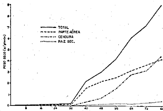
Fig. 1. Peso de matéria seca encontrado em diversas épocas após a germinação.
