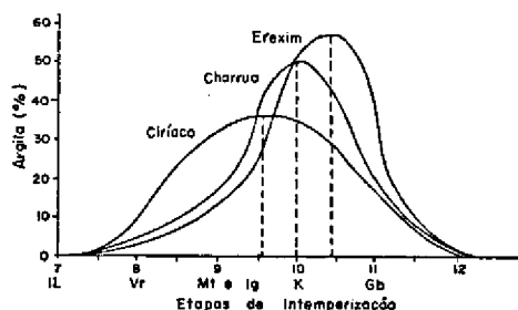
FIG. 8. Curvas de distribuição de freqüência das argilas nas várias etapas de intemperização: IL = illita; Mt = montmorilonita; K = caulinita e haloisita; Vr = vermiculita; Gb = gibbrite e materiais amorfos; Ig = minerais inter-estratificados. 2:1 e 2:2.
