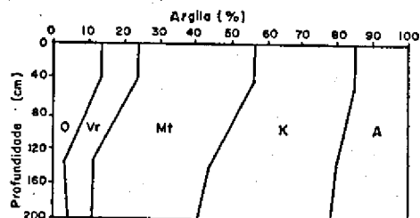
FIG. 7. Composição mineralógica da fração argila do solo Ciriaco; A = materiais amorfos; K = caulinita + haloisita; Mt = montmorilonita; Vr = vermiculita; O = outros, como feldspatos, micas, etc.
