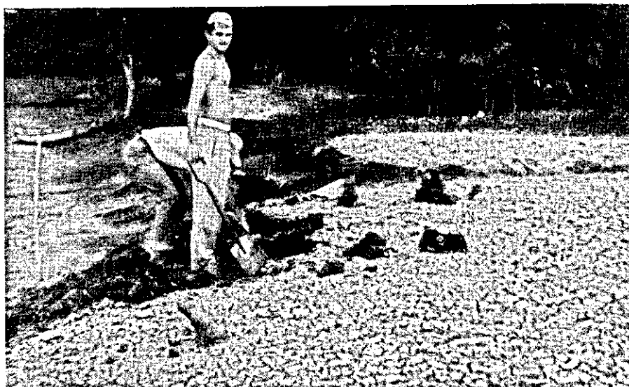
FIG. 27. Aspecto de um solo Hidromórfico quando seco. Note-se a camada superficial com pequenas rachaduras. Ao fundo, vegetação de mangue.
