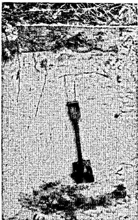
FIG. 21. Perfil de Regosol. Estrada de Sta. Maria-S. Miguel do Guamá.
