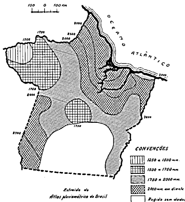
FIG. 1. Isoetas anuais do Estado do Pará e do Território Federal do Amapá.
