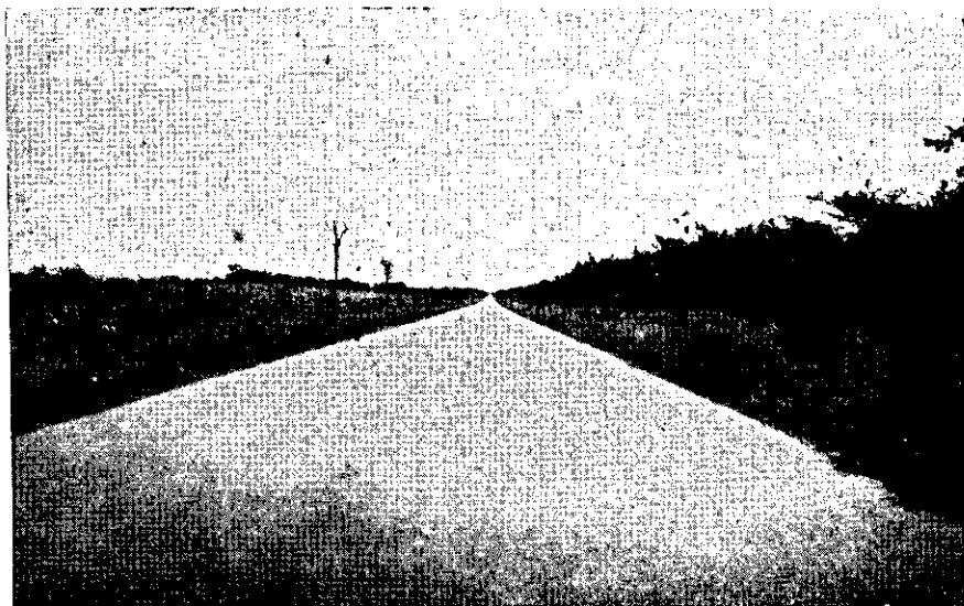
FIG. 2. Aspecto do relevo geral do Latosol Amarelo, Região Bragantina.
