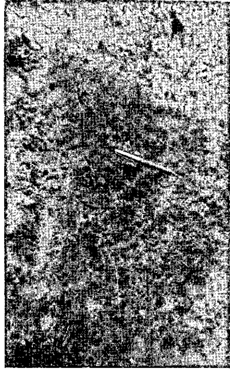
FIG 16. Latosol Concrecionário, observando-se ocorrência abundante de concreções lateríticas.
