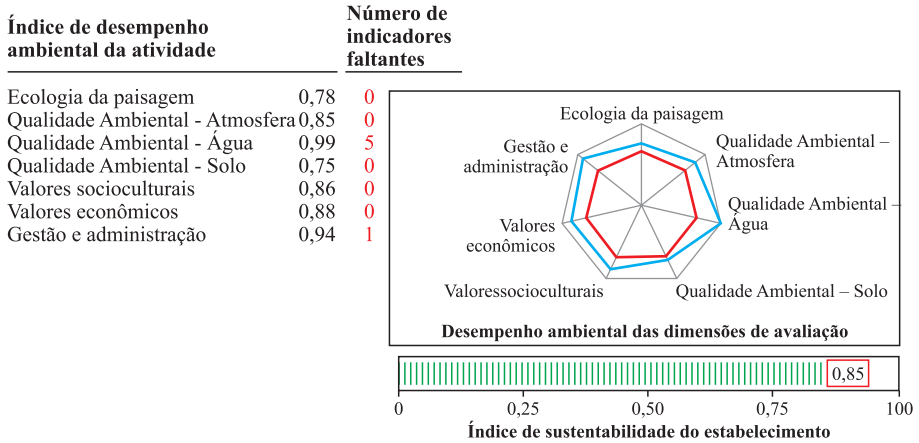
Figura 2. Desempenho ambiental e índice integrado de sustentabilidade observados na Chácara Vale Verde, segundo as dimensões de avaliação do sistema de indicadores Apoiar-NovoRural, em maio de 2017.
