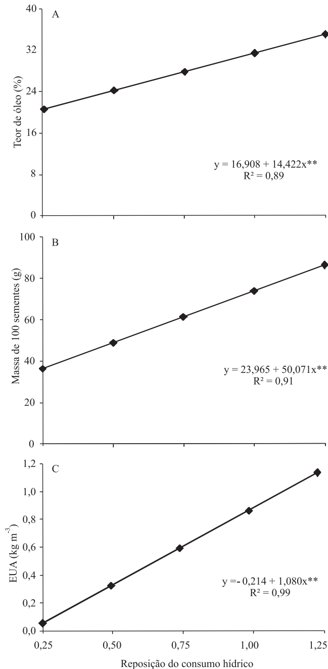
Figura 1. A, teor de óleo; B, massa de 100 sementes; e C, eficiência do uso da água (EUA) de sementes de pinhão manso em razão da reposição hídrica com água residuária.
