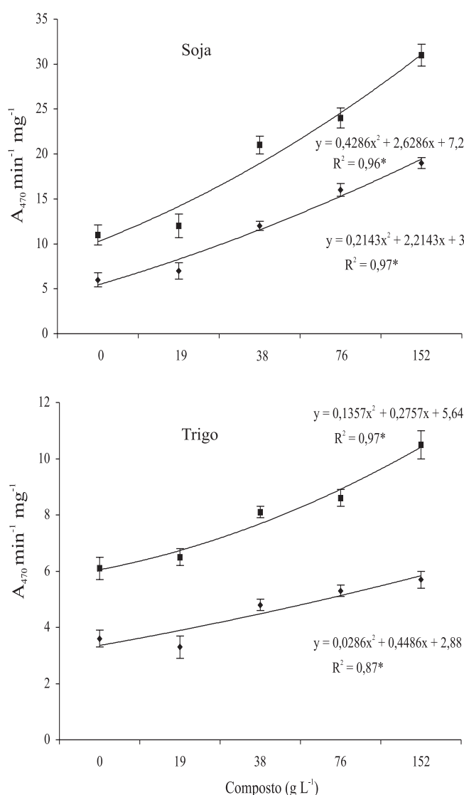
Figura 2. Atividade da peroxidase nas folhas (◆) e nas raízes (■) de plântulas de soja e trigo submetidas a concentrações crescentes de extrato do composto de lodo têtil.
