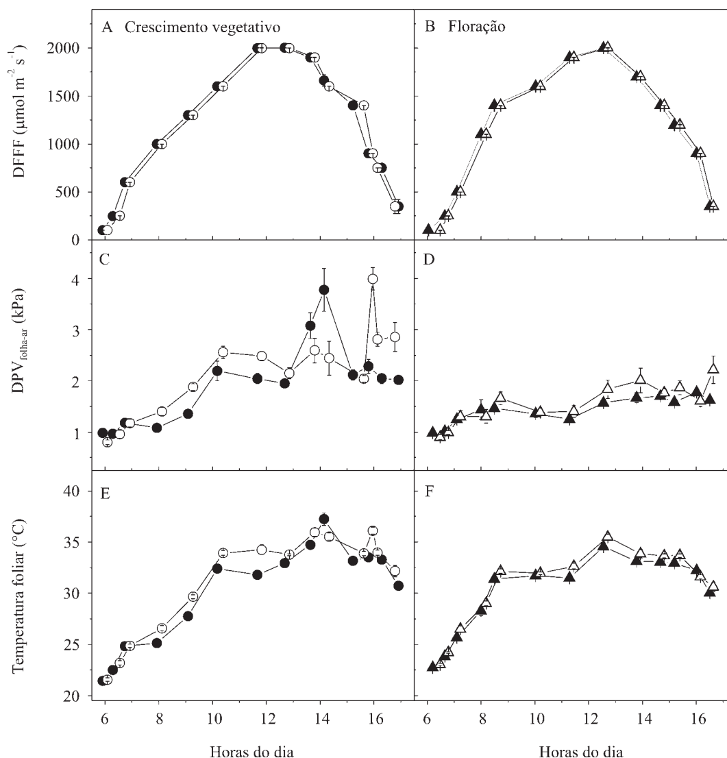
Figura 1. Curso diário da densidade de fluxo de fótons fotossinteticamente ativos (DFFF), da diferença de pressão de vapor entre a folha e o ar (DPV folha-ar ) e da temperatura foliar, nas cultivares de amendoim Runner IAC-886 (símbolos cheios) e IAC-Caiapó (símbolos vazios), no estágio vegetativo (●, ○) e em plena floração (▲, △), sob condições naturais. Cada ponto representa o valor médio ( \pm erro-padrão) de cinco repetições, em plantas diferentes.
