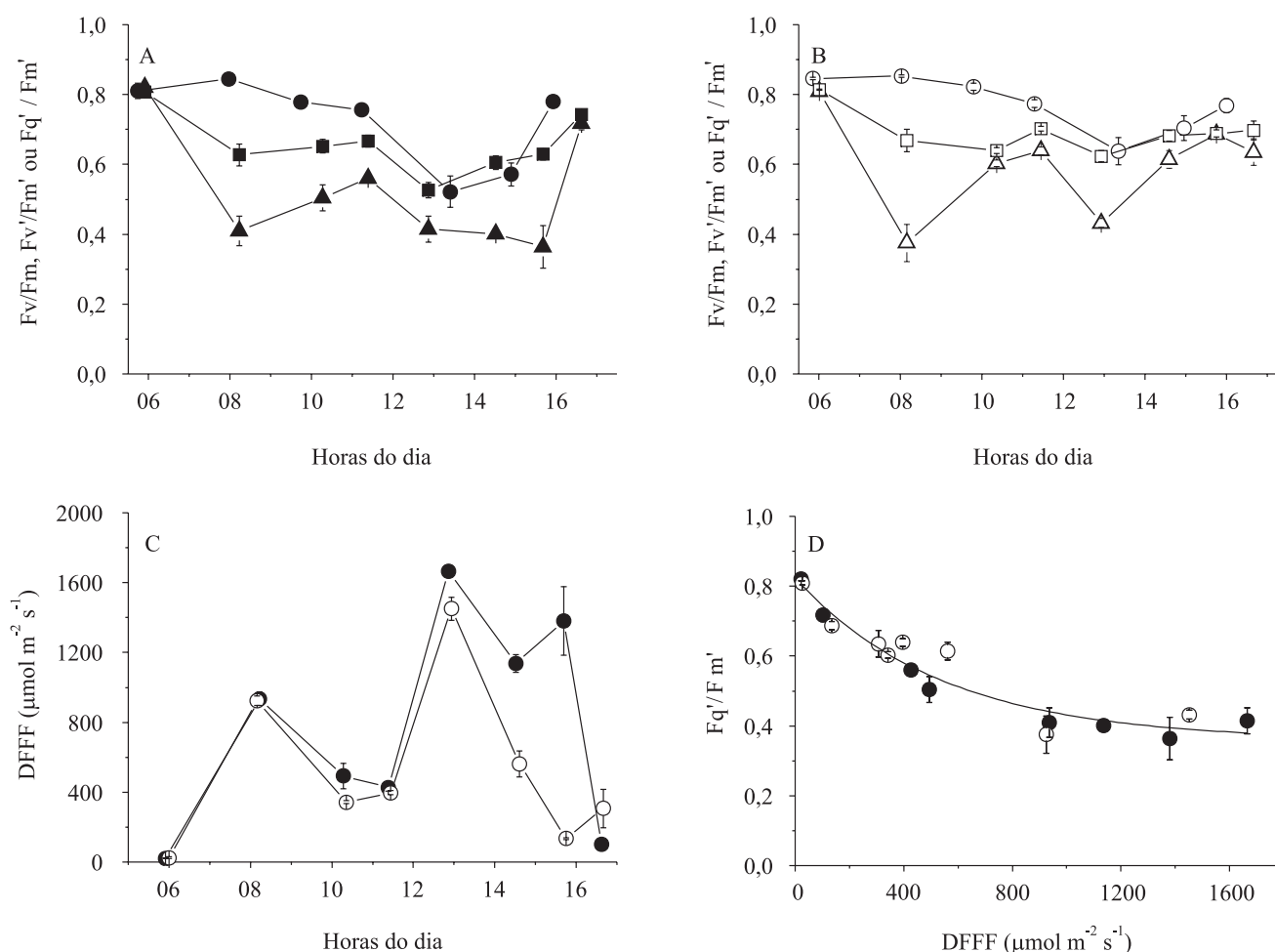
Figura 6. Curso diário da eficiência quântica máxima ( F_v/F_m : ● em A, ○ em B), da eficiência máxima ( F_v'/F_m' : ■, □) e da eficiência operacional ( F_q'/F_m' : ▲, △) do FSII, e densidade de fluxo de fótons fotossinteticamente ativos (DFFF) da radiação solar (C) registrada durante as medidas, nas cultivares de amendoim Runner IAC-886 (A e símbolos cheios) e IAC-Caiapó (B e símbolos vazios), sob condições naturais. Em D, eficiência operacional ( F_q'/F_m' ) do FSII em função da DFFF. Cada ponto representa o valor médio ( \pm erro-padrão) de seis repetições, em plantas diferentes.
