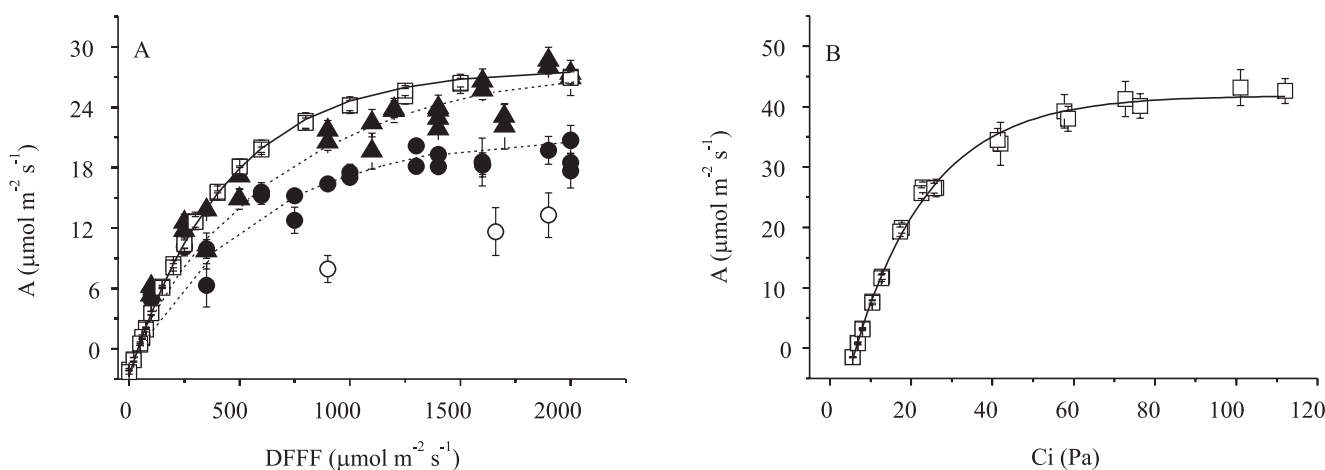
Figura 5. Taxa de assimilação líquida de \text{CO}_2 ( A ) em função da densidade de fluxo de fótons fotossinteticamente ativos (DFFF) e da concentração interna de \text{CO}_2 ( C_i ), nas cultivares de amendoim, sob condições controladas (□) e sob condições naturais, no estágio vegetativo (●) e de florescimento (▲). Os pontos obtidos com \text{DPV}_{\text{folha-ar}} maior que 3,0 estão indicados (○). Cada ponto representa o valor médio de cinco (●, ○, ▲) ou de quatro (□) repetições ( \pm erro-padrão), em plantas diferentes.
