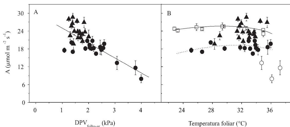
Figura 4. Taxa de assimilação líquida de \text{CO}_2 ( A ) em função da diferença de pressão de vapor entre a folha e o ar ( \text{DPV}_{\text{folha-ar}} ) e da temperatura da folha, nas cultivares de amendoim, no estágio vegetativo (●) e de florescimento (▲). Os pontos obtidos em \text{DPV}_{\text{folha-ar}} maior que 3,0 (○) e as medidas realizadas em condições controladas (□) estão indicados. Cada ponto representa o valor médio de cinco (●, ○, ▲) ou de três (□) repetições ( \pm erro-padrão), em plantas diferentes.
