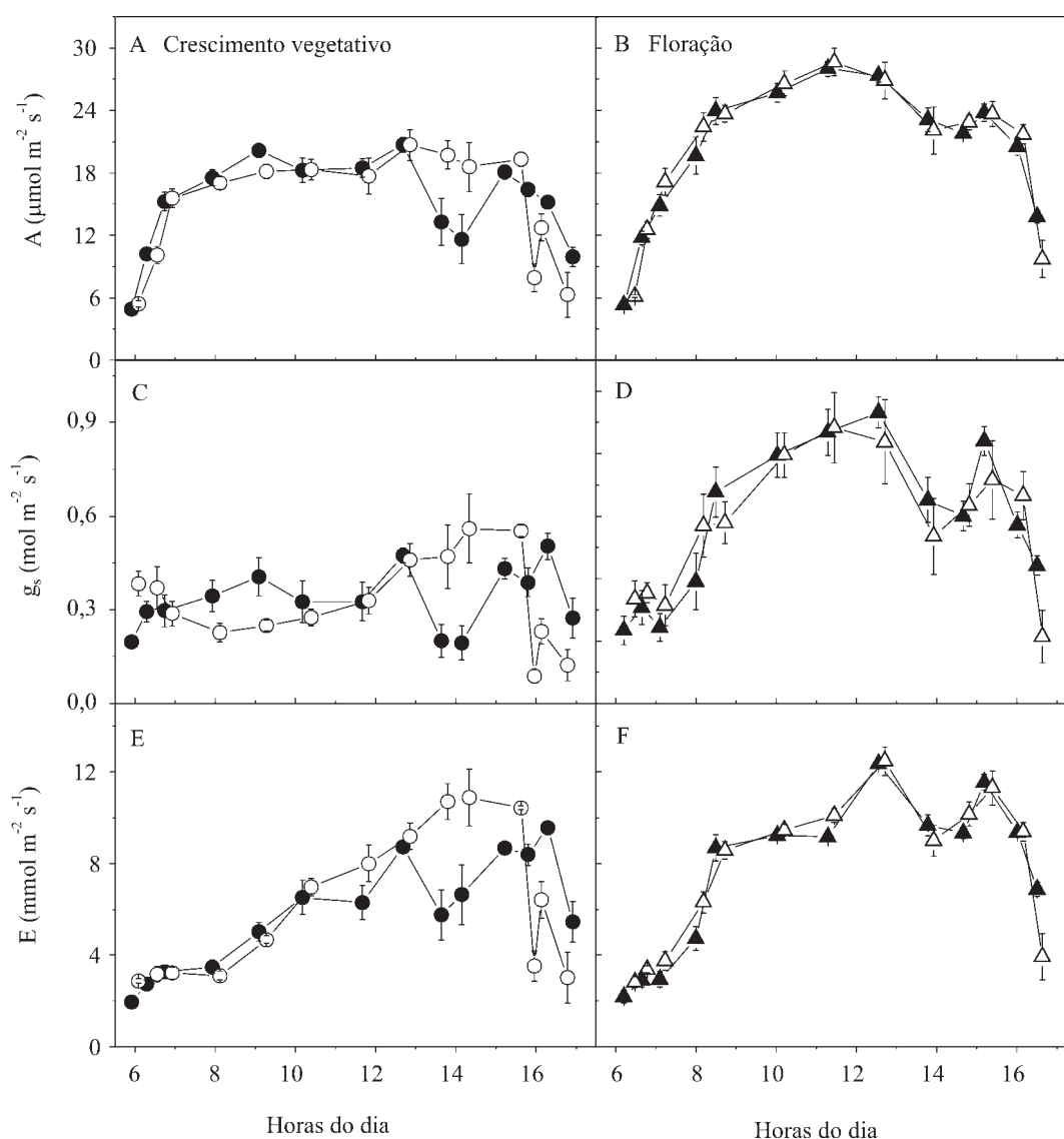
Figura 2. Curso diário da taxa de assimilação líquida de CO 2 (A), condutância estomática ( g_s ) e da taxa de transpiração (E) nas cultivares de amendoim Runner IAC-886 (símbolos cheios) e IAC-Caiapó (símbolos vazios), no estágio vegetativo (●, ○) e em plena floração (▲, △). Cada ponto representa o valor médio ( \pm erro-padrão) de cinco repetições, em plantas diferentes.
