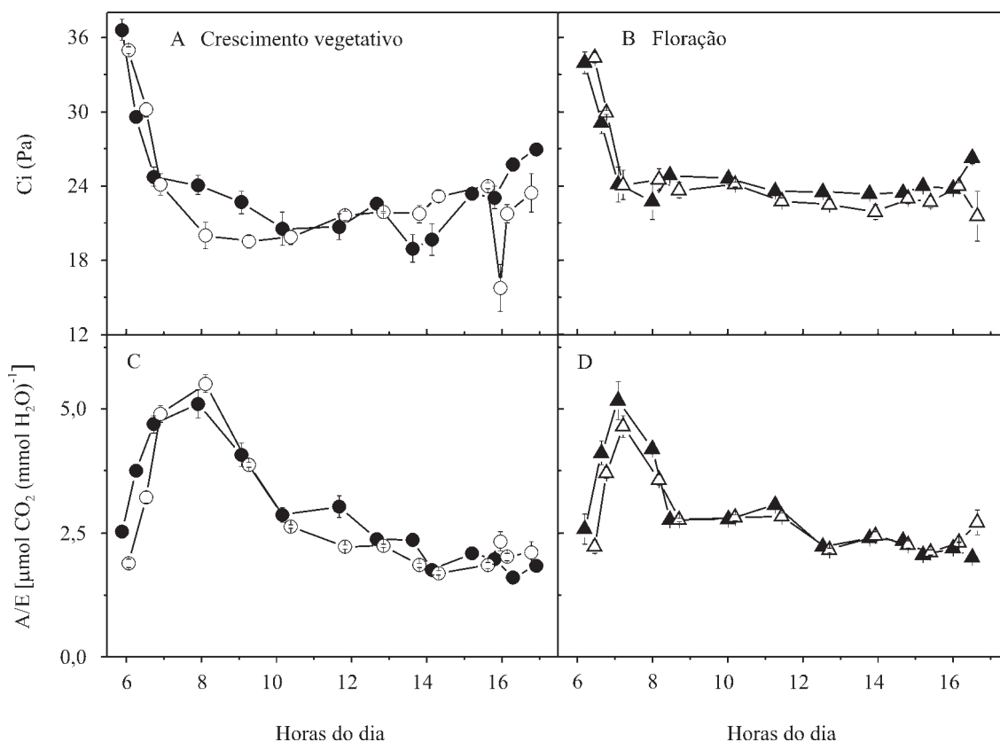
Figura 3. Curso diário da concentração interna de \text{CO}_2 ( C_i ) e da eficiência do uso da água ( A/E ), nas cultivares de amendoim Runner IAC-886 (símbolos cheios) e IAC-Caiapó (símbolos vazios), no estágio vegetativo (●, ○) e em plena floração (▲, △). Cada ponto representa o valor médio ( \pm erro-padrão) de cinco repetições, em plantas diferentes.
